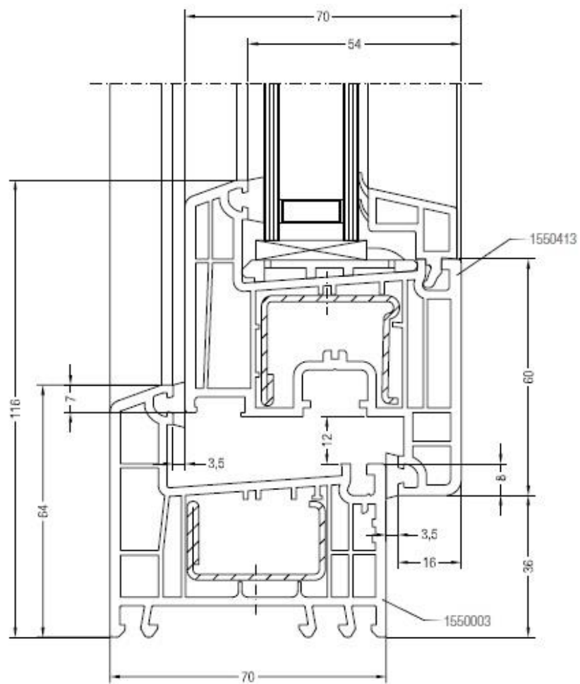
Sezione nodo anta dritta
